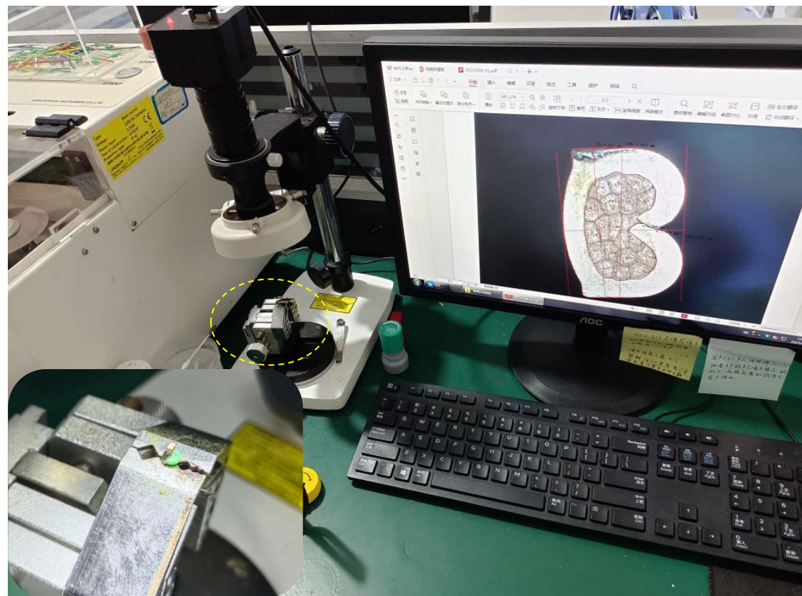
导线与端子压接截面分析
