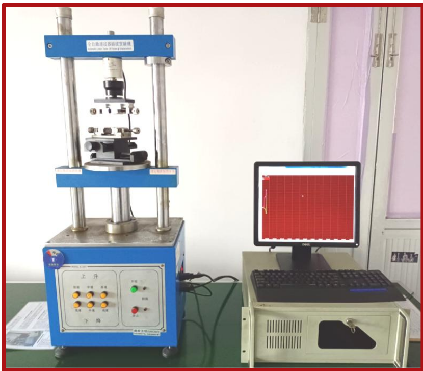
Automatic Linker Tester Of Forces&Displacement 全自动连接器插拔试验机
